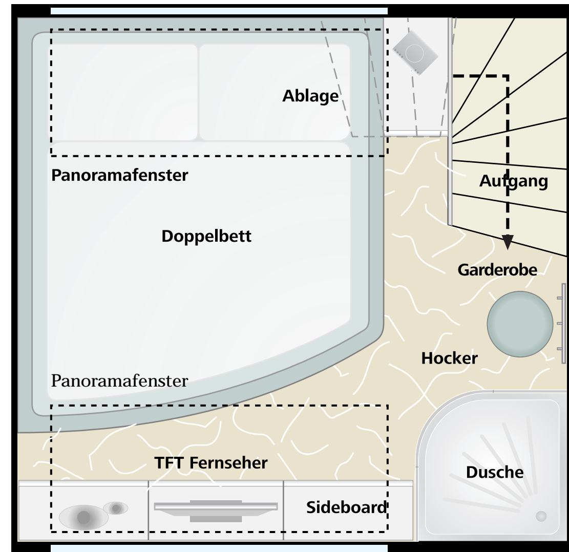
Draufsicht Erdgeschoss
